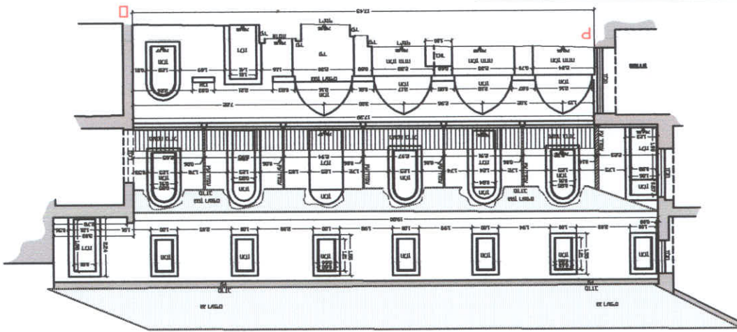
חיתוך P-Q (פס 17 צד דרום)
