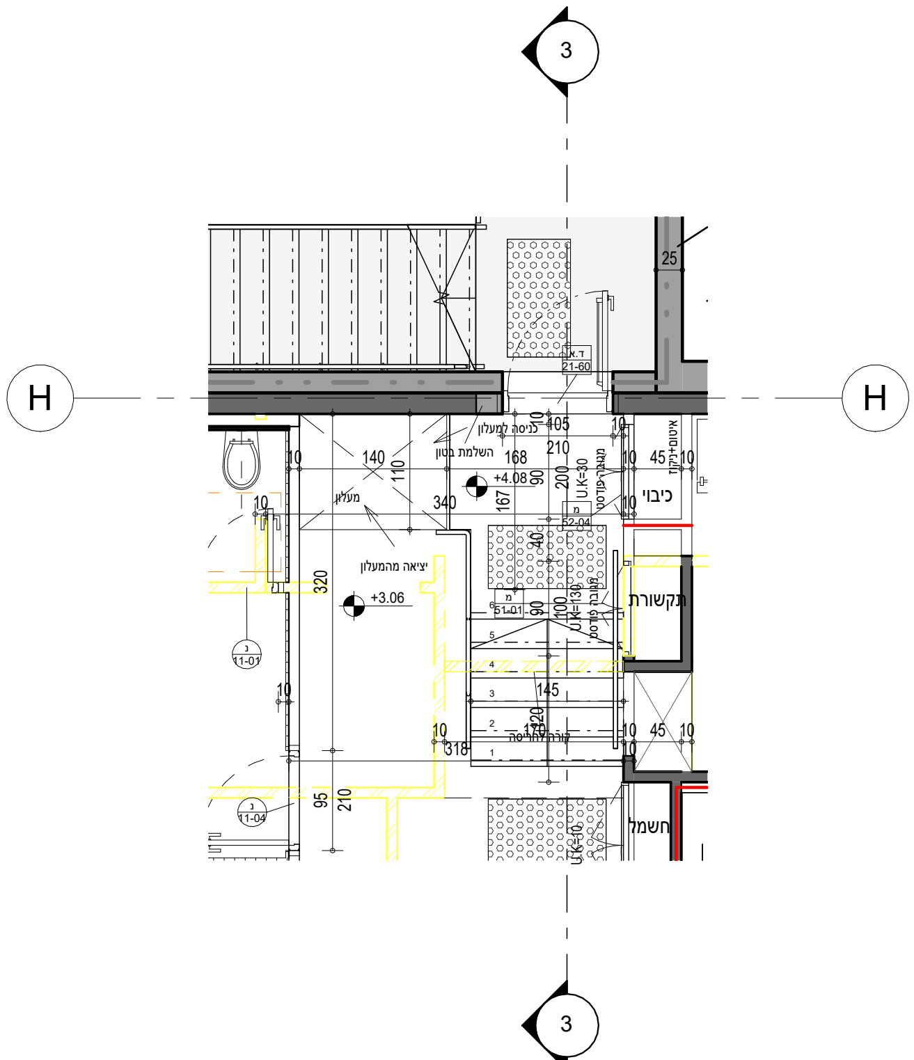
תוכנית קומה 1 מבנה משרדים קנ"מ: 1 : 50 1 R-07
