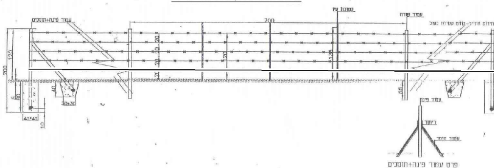
מפרט לגדר בקר 5 חוטי תייל
