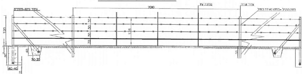
מפרט לגדר בקר 4 חוטי תייל
