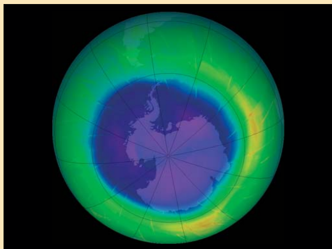
החור בשכבת האוזון (בכחול) במצבו בספטמבר 2009
